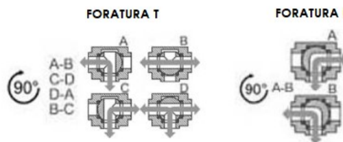
Valvola a sfera a 3 vie e 4 guarnizioni con foratura sfera a "T" o "L" da definire in fase di richiesta
