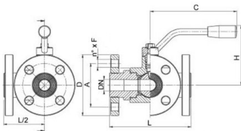
Valvola a sfera a 3 vie e 4 guarnizioni con foratura sfera a "T" o "L" da definire in fase di richiesta
