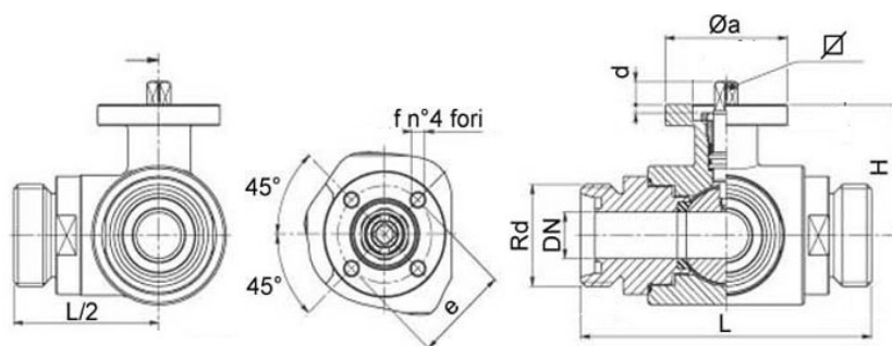
Valvola a sfera a 3 vie e 4 guarnizioni con foratura sfera a "T" o "L" da definire in fase di richiesta
