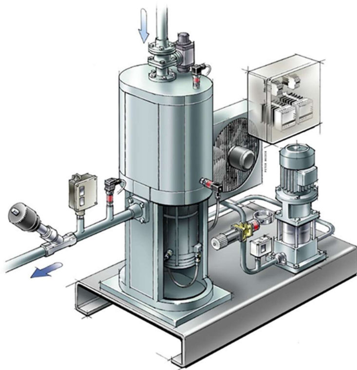
Applicazione tipo per sensori di pressione e temperatura
