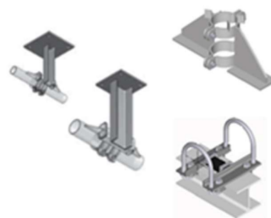
esempio di punto fisso
