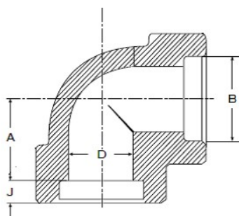
GOMITO 90° Elbows
