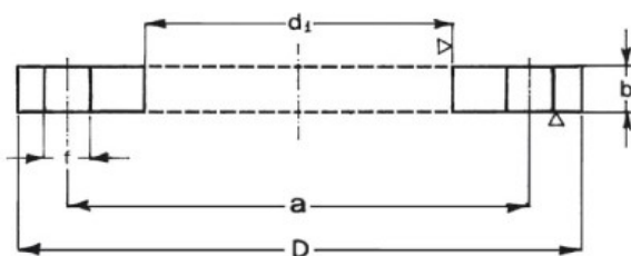
Flange piane A105 EN1092-1-01
