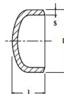
FONDELLI Caps
