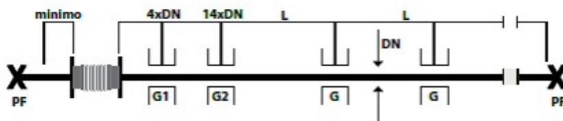
Esempio di tubazione non guidata
